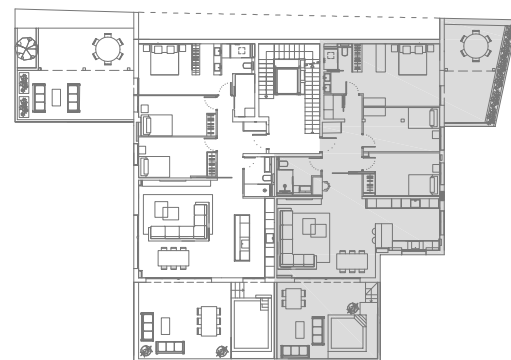
PLANTA SEGONA
