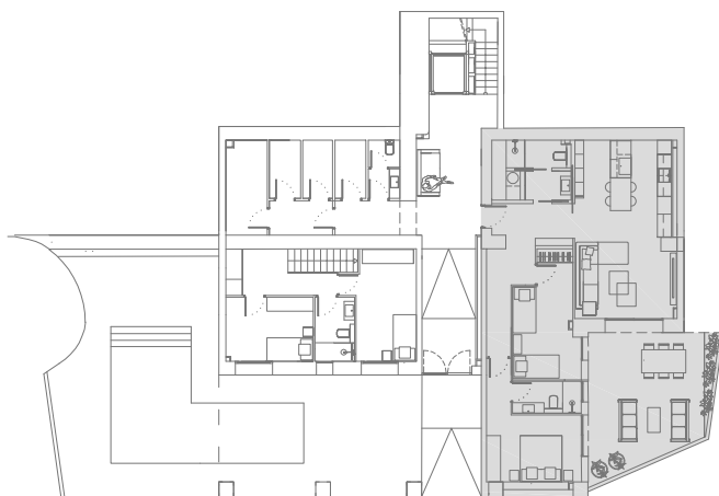
PLANTA BAIXA
