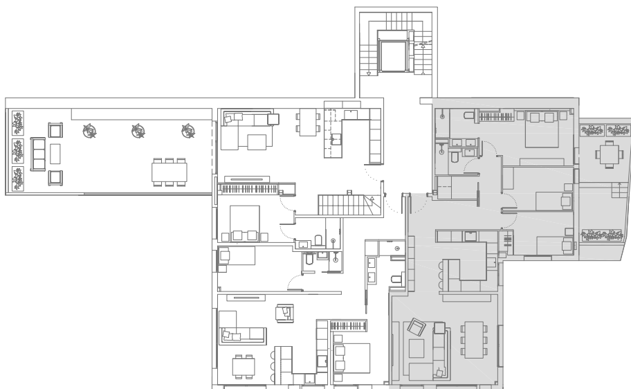
PLANTA PRIMERA
