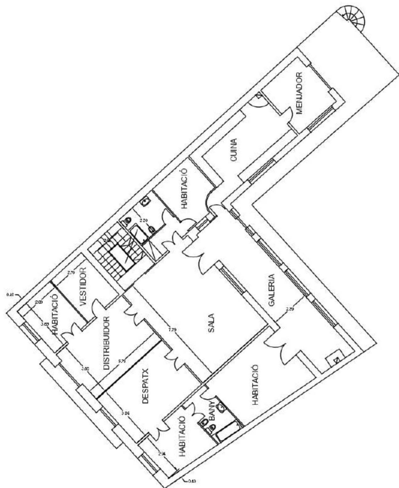
PLANTA PRIMERA
